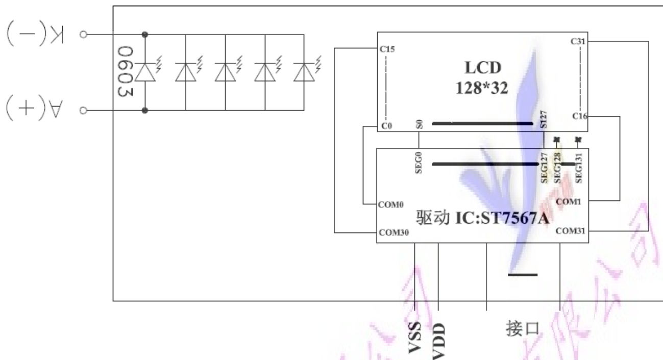
图2:COG12832TM550图像点阵型液晶模块的电路框图
