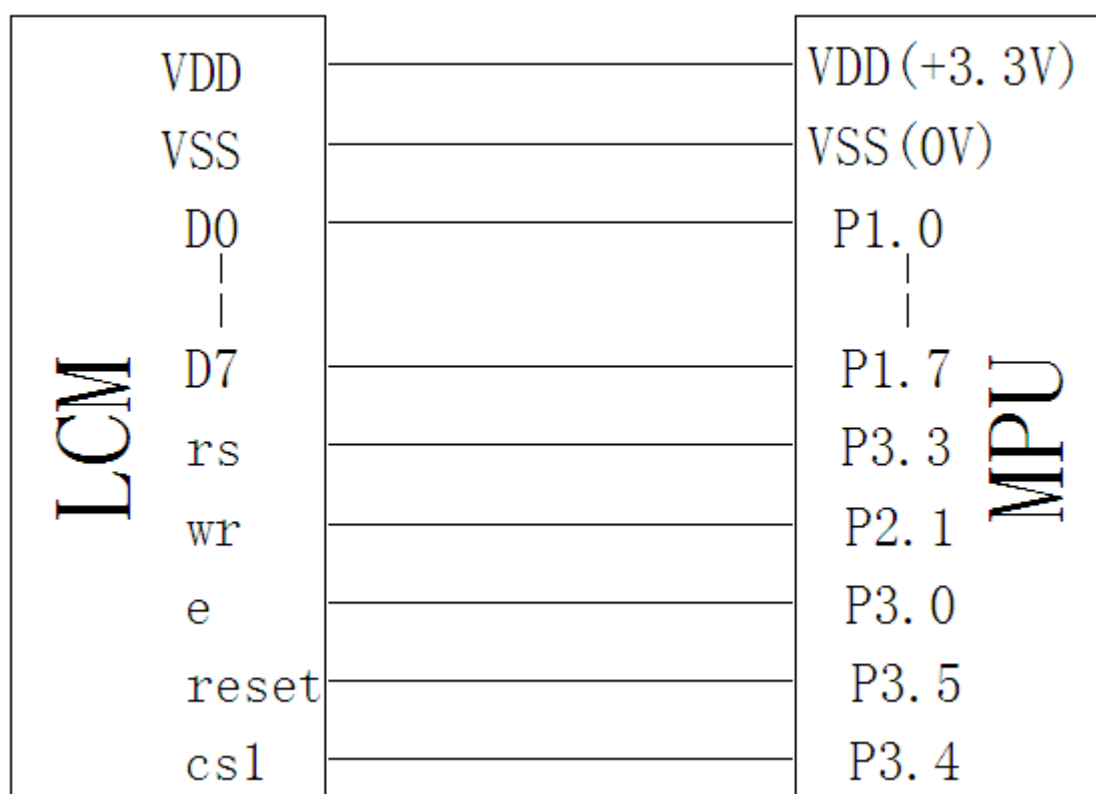
图 9. 并行接口
